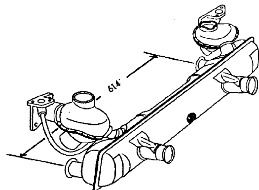
113 251 053 AJ mit Wärmetauschern 2 Anschlüsse für Endrohre
