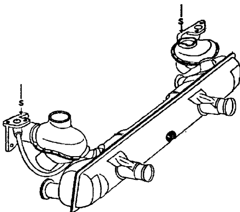
111 251 053 mit Wärmetauschern, 2 Anschlüsse für Endrohre auf den Flanschen mit „S“ gezeichnet
