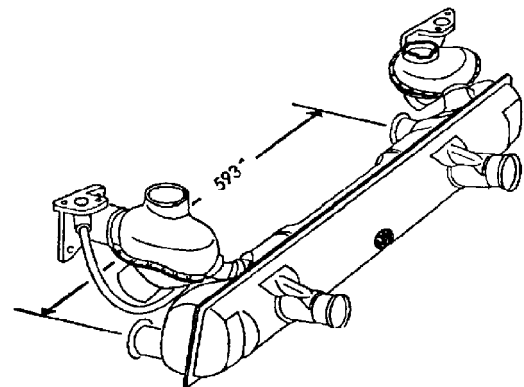
113 251 053 L mit Wärmetauschern 2 Anschlüsse für Endrohre
