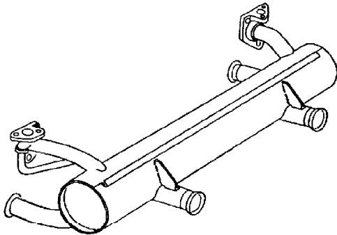
111 251 051 G ohne Wärmetauscher 2 Anschlüsse für Endrohre
